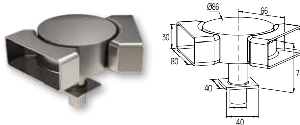
ΣΥΝΔΕΣΜΟΣ ΜΕΤΑΒΛΗΤΗΣ ΓΩΝΙΑΣ ΚΟΥΠΑΣΤΗΣ 80x30 ΜΕ ΚΟΛΩΝΑ F50-102 ADJUSTABLE CORNER CONNECTOR FOR 80x30 HANDRAIL WITH F50-102 COLUMN Κωδ. / Code 4357
