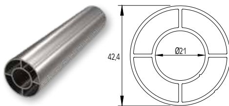
ΚΟΛΩΝΑ ΣΤΗΡΙΞΗΣ Ø42 SUPPORT COLUMN Ø42 Κωδ. / Code F50-100 Βάρος / Weight 1025 gr/m
