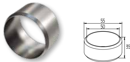
ΣΥΝΔΕΣΜΟΣ ΚΟΥΠΙΑΣΤΩΝ Ø50 CONNECTOR FOR HANDRAIL Ø50
