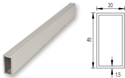
ΠΡΟΦΙΛ 40x20 PROFILE 40x20
