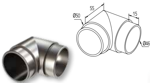
ΣΥΝΔΕΣΜΟΣ 90° ΓΙΑ ΚΟΥΠΑΣΤΗ \varnothing 50 CONNECTOR 90° FOR HANDRAIL \varnothing 50
