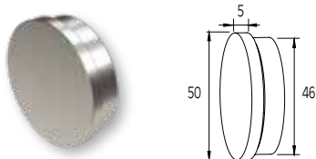
ΤΑΠΑ ΚΟΥΠΑΣΤΗΣ F50-200 (ΕΠΙΠΕΔΗ) END CAP FOR F50-200 HANDRAIL (FLAT)
