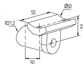
ΕΞΩΤΕΡΙΚΟ ΣΤΗΡΙΓΜΑ ΚΟΥΠΑΣΤΗΣ Ø50 ΜΕ ΚΟΛΩΝΑ Ø42 EXTERNAL SUPPORT FOR HANDRAIL Ø50 WITH COLUMN Ø42
