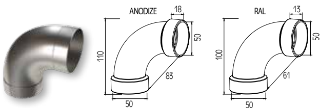
ΓΩΝΙΑΚΟΣ ΣΥΝΔΕΣΜΟΣ 90° ΚΟΥΠΙΑΣΤΩΝ Ø50 CONNECTOR 90° FOR HANDRAIL Ø50
