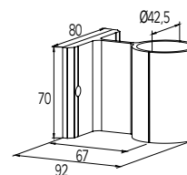
ΕΞΩΤΕΡΙΚΟ ΣΤΗΡΙΓΜΑ ΓΙΑ ΚΟΛΩΝΑ Ø42 EXTERNAL SUPPORT FOR Ø42 COLUMN
