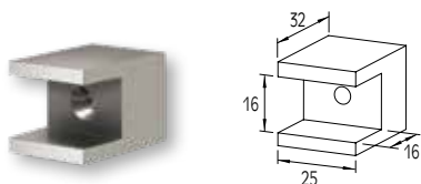
ΣΥΝΔΕΣΜΟΣ ΚΟΛΩΝΑΣ F50-102/106 ΜΕ ΠΡΟΦΙΛ F50-302 CONNECTOR FOR F50-102/106 COLUMN WITH PROFILE F50-302
