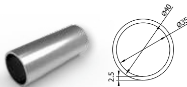
ΚΟΥΡΠΑΣΤΗ Ø40 HANDRAIL Ø40
