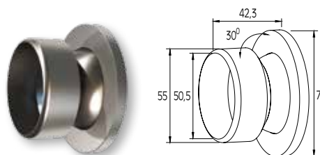
ΑΡΜΟΚΑΛΥΠΤΡΟ ΚΟΥΠΑΣΤΗΣ Ø50 (ΜΕ ΚΑΠΑΚΙ) WALL COVER FOR HANDRAIL Ø50 WITH CAP
