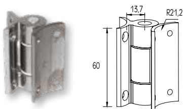
ΜΕΝΤΕΣΣ ΚΟΛΩΝΑΣ F50-100 HINGE FOR F50-100 COLUMN
