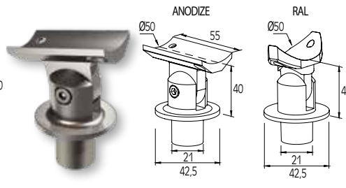
ΣΥΝΔΕΣΜΟΣ ΚΟΥΠΑΣΤΗΣ Ø50 ΜΕ ΚΟΛΩΝΑ Ø42 (ΣΚΑΛΑ) CONNECTOR FOR HANDRAIL Ø50 WITH COLUMN Ø42 (STAIRS)
