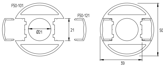
ΚΑΠΑΚΙ ΓΙΑ ΚΟΛΩΝΑ/ΚΟΥΠΑΣΤΗ F50-101 COVER FOR COLUMN/HANDRAIL F50-101 Κωδ. / Code F50-121 Βάρος / Weight 152 gr/m
