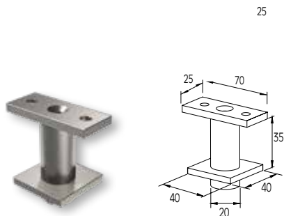
ΣΤΗΡΙΓΜΑ ΚΟΛΩΝΑΣ F50-102 ΜΕ ΚΟΥΠΑΣΤΗ F50-201 SUPPORT FOR F50-102 COLUMN WITH F50-201 HANDRAIL
