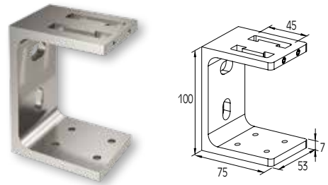
ΕΞΩΤΕΡΙΚΟ ΣΤΗΡΙΓΜΑ ΚΟΛΩΝΑΣ BLADE EXTERNAL SUPPORT FOR BLADE COLUMN Κωδ. / Code 4142
