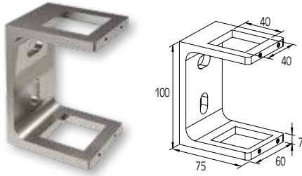
ΕΞΩΤΕΡΙΚΟ ΣΤΗΡΙΓΜΑ ΚΟΛΩΝΑΣ 40x40 EXTERNAL SUPPORT FOR 40x40 COLUMN Κωδ. / Code 4139
