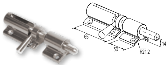
ΣΥΡΤΗΣ ΚΟΛΩΝΑΣ F50-100 BOLT FOR F50-100 COLUMN
