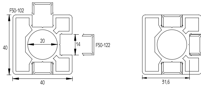
ΚΑΠΑΚΙ ΚΟΛΩΝΑΣ F50-102 COVER FOR F50-102 COLUMN Κωδ. / Code F50-122 Βάρος / Weight 86 gr/m
