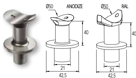
ΣΥΝΔΕΣΜΟΣ ΚΟΥΠΑΣΤΗΣ Ø50 ΜΕ ΚΟΛΩΝΑ Ø42 CONNECTOR FOR HANDRAIL Ø50 WITH COLUMN Ø42
