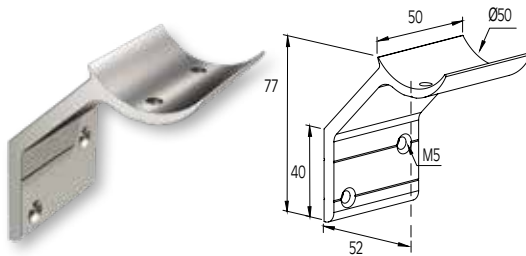
ΕΠΙΤΟΙΧΙΟ ΣΤΑΘΕΡΟ ΣΤΗΡΙΓΜΑ ΚΟΥΠΑΣΤΗΣ F50-200 FIXED WALL SUPPORT FOR F50-200 HANDRAIL Κωδ. / Code 4141
