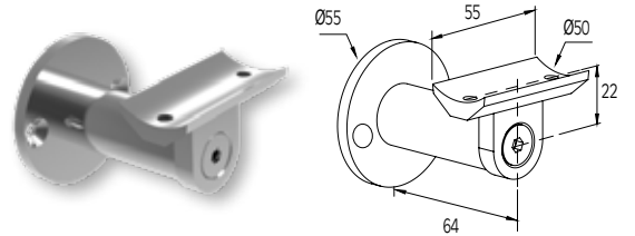
ΕΠΙΤΟΙΧΙΟ ΣΤΗΡΙΓΜΑ ΚΟΥΠΑΣΤΗΣ F50-200 WALL SUPPORT FOR F50-200 HANDRAIL Κωδ. / Code 4140
