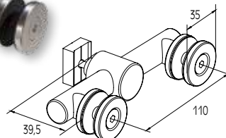
ΣΤΗΡΙΓΜΑ ΤΖΑΜΙΟΥ ΔΙΠΛΟ 8-10mm ΓΙΑ ΚΟΛΩΝΑ BLADE SINGLE GLASS SUPPORT 8-10mm FOR BLADE COLUMN
