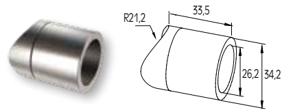
ΣΥΝΔΕΣΜΟΣ ΚΟΛΩΝΑΣ F50-100 ΜΕ ΠΡΟΦΙΛ \varnothing 26 CONNECTOR FOR F50-100 COLUMN WITH PROFILE \varnothing 26
