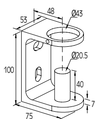
ΕΞΩΤΕΡΙΚΟ ΣΤΗΡΙΓΜΑ ΚΟΛΩΝΑΣ F50-100/103 EXTERNAL SUPPORT FOR F50-100/103 COLUMN
