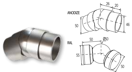
ΣΥΝΔΕΣΜΟΣ ΜΕΤΑΒΛΗΤΗΣ ΓΩΝΙΑΣ ΚΟΥΠΑΣΤΩΝ Ø50 ADJUSTABLE CORNER CONNECTOR FOR COLUMN Ø50
